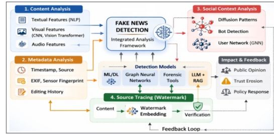
Hình 1. Khung phát hiện tin giả đa tầng trong kỷ nguyên AI tạo sinh
