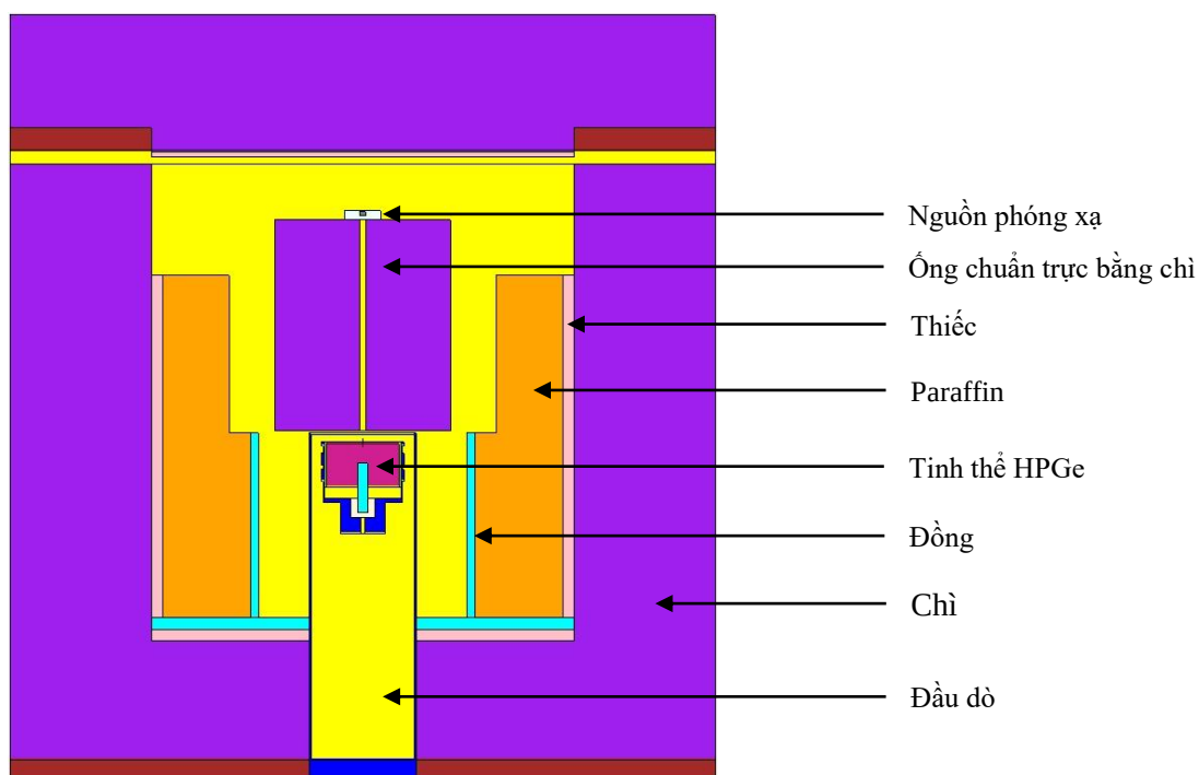
Hình 1. Mặt cắt đứng của buồng đo phổ gamma với nguồn phóng xạ và ống chuẩn trực điển hình vẽ bằng chương trình MCNP4C2. Trường hợp nguồn đặt cách dầu dò 15 cm, ống chuẩn trực bằng chì bán kính khẩu độ 0,25 cm và bán kính ngoài 5,35 cm.
