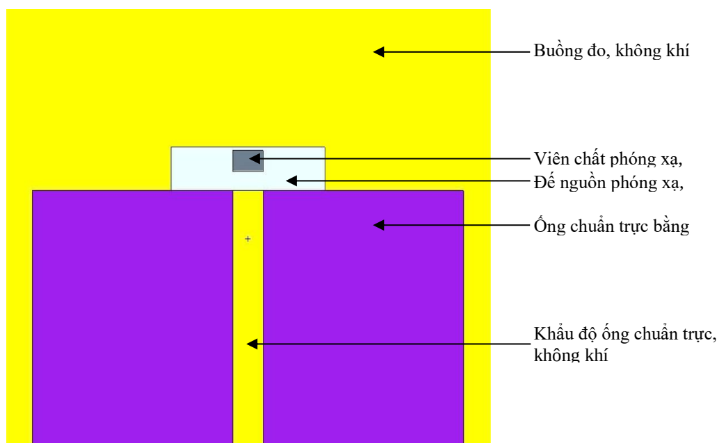
Hình 2. Mặt cắt đứng của nguồn phóng xạ vẽ bằng chương trình máy tính mô phỏng Monte Carlo MCNP4C2. Cấu trúc và kích thước hình học do hãng Eckert & Ziegler,
