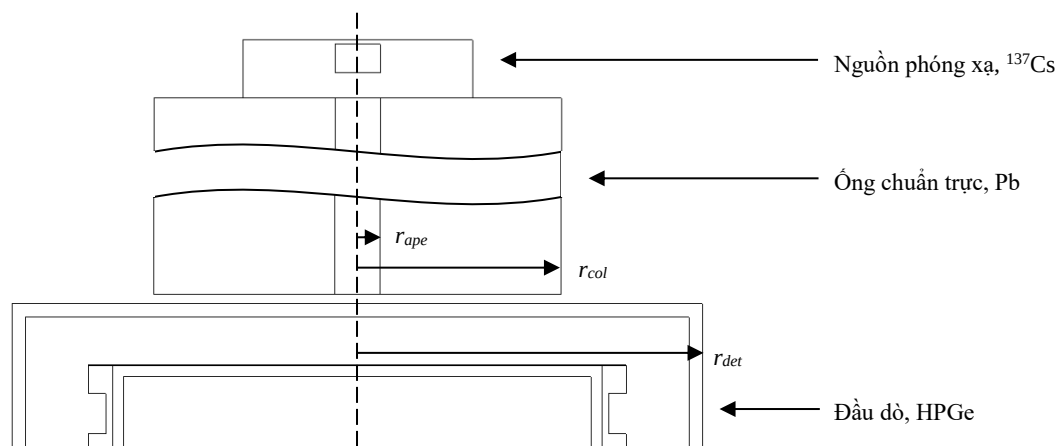
Hình 3. Ống chuẩn trực cùng với nguồn phóng xạ và đầu dò được bố trí đồng trục với nhau. Trong đó: r_{ape} , r_{col} và r_{det} lần lượt là bán kính khẩu độ, bán kính ống chuẩn trực và bán kính đầu dò.
