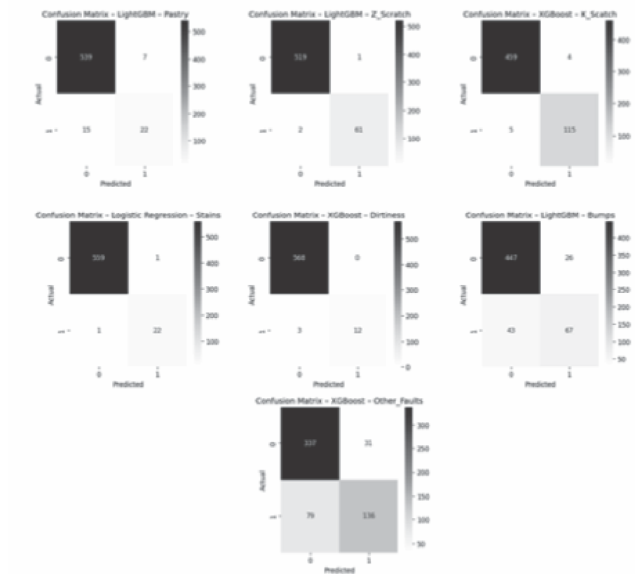
Hình 2. Kết quả ma trận nhầm lẫn đối với 7 lỗi
