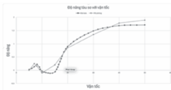
Hình 5. Đồ thị độ nâng so với vận tốc
