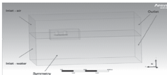
Hình 3. Điều kiện biên
