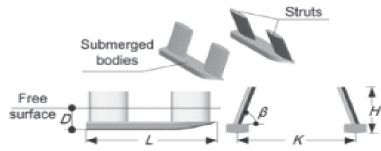
Hình 1. Sơ đồ mô hình tàu hai thân
