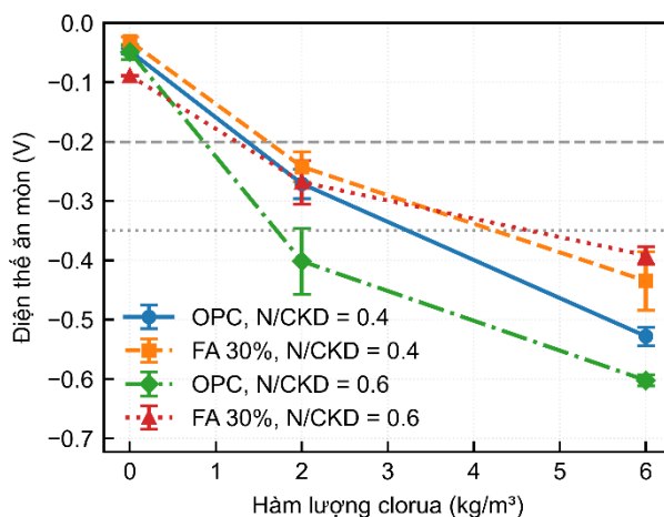
Hình 2. Quan hệ giữa điện thế ăn mòn và hàm lượng clorua trong các cấp phối bê tông sau 365 ngày.
