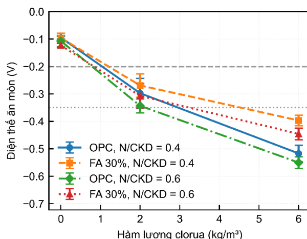
Hình 1. Quan hệ giữa điện thế ăn mòn và hàm lượng clorua trong các cấp phối bê tông sau 150 ngày.
