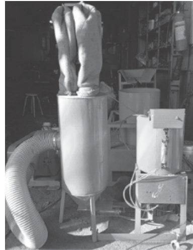
Hình 7. Hình ảnh thiết bị lọc tách bột rơm rạ và máy trộn rơm rạ sau khi chế tạo
