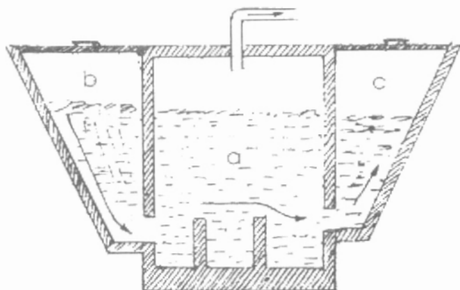
Sơ đồ cắt dọc bể khí sinh vật
