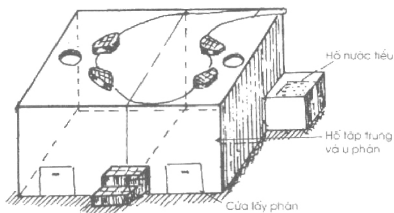
Hình 16. Nhà tiêu 2 ngăn ủ phân tại chỗ
