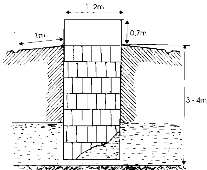
Hình 6b. Sơ đồ giếng khơi xây khẩu
