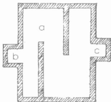
Sơ đồ cắt ngang bể khí sinh vật
