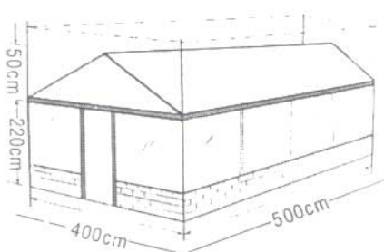
Mô hình nhà kính trồng lan kết cấu bằng kính và hợp kim nhôm khép kín hoàn toàn
