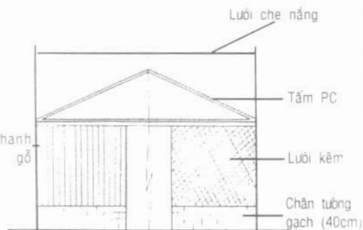
Mô hình nhà trồng lan đơn giản kết cấu bằng gỗ.
