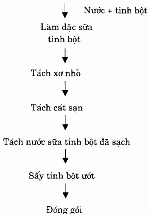
Hình 11. Sơ đồ sản xuất tinh bột khoai tây (công nghiệp)
