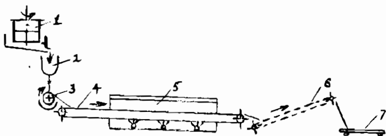
Hình 14. Sơ đồ cơ giới hóa sản xuất bánh trắng
