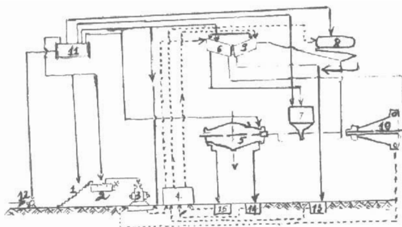
Hình 15. Sơ đồ kỹ thuật sản xuất tinh bột bằng cơ giới
