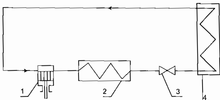
Hình 3. Sơ đồ hệ thống máy lạnh
