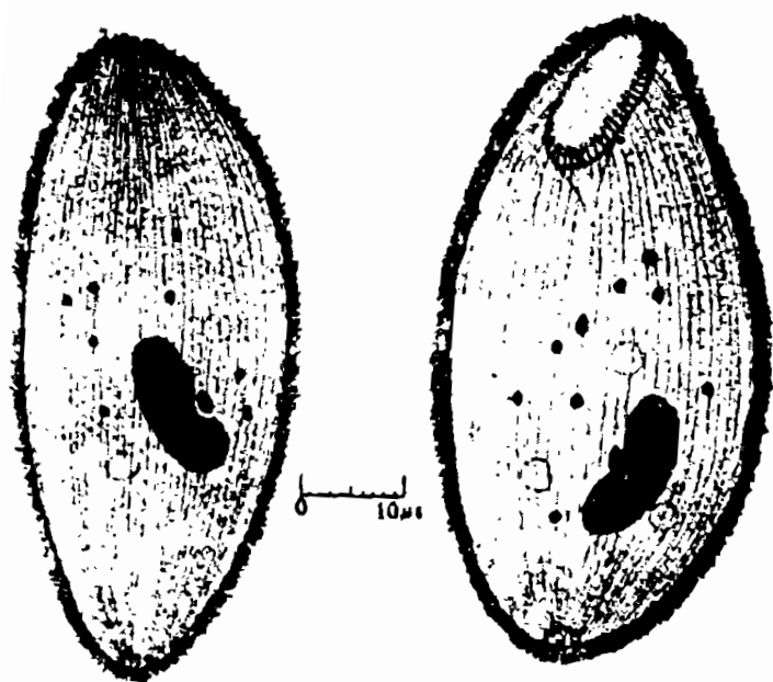
Hình 35: Balantidium ctenopharyngodoni
