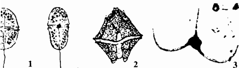
Hình 61: Tảo giáp
