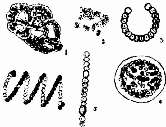
Hình 59: Mycrocystis
