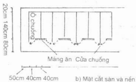
b) Mặt cắt sàn và nền
