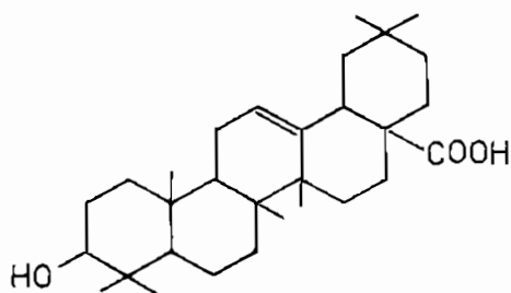
3- Hydroxy -[12] - olean [28] ovic acid
