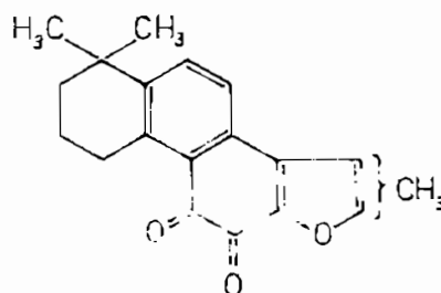
Tansinon II
