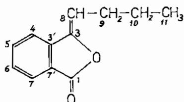
Ligustilid
