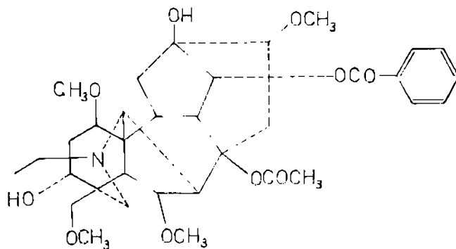
Aconitin
