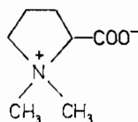
Stachydrin
