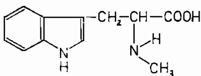
Abrin C 12 H 14 N 2 O 2
