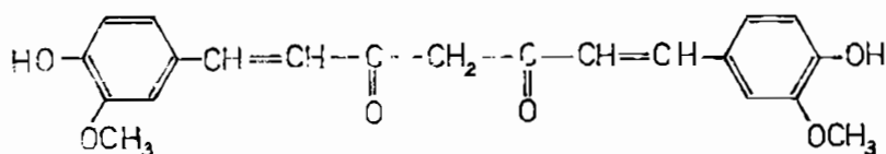
Curcumin
