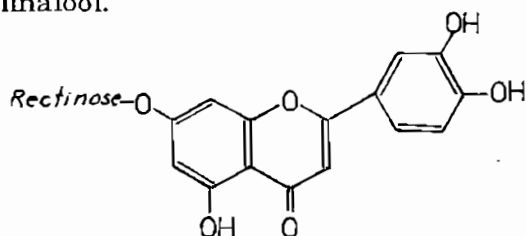
Scolymosid
