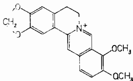
Berberin
