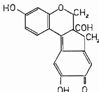
Brasilein
