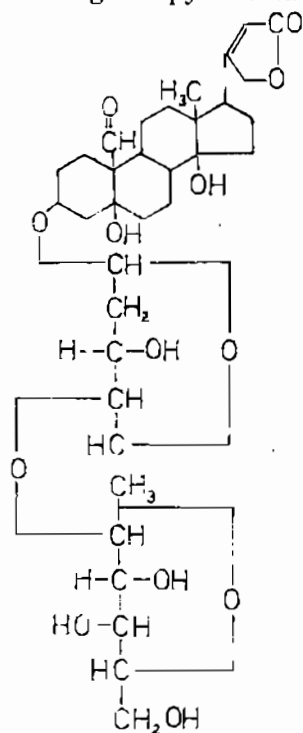
Olitorisid
