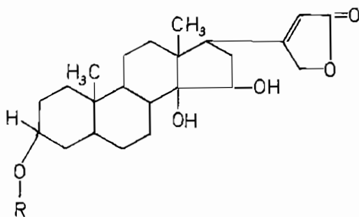
Rodesin B = R là L - rhamnoza
