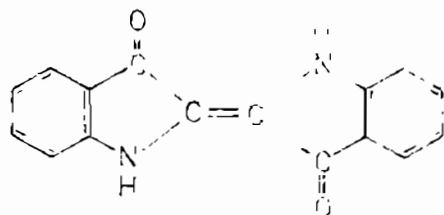
Indigotin (màu sẫm)
