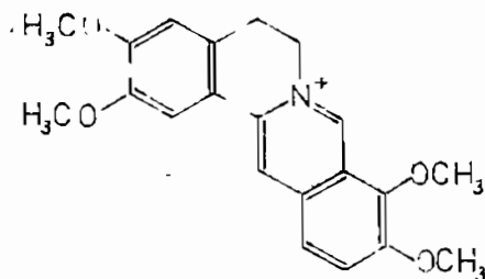
Palmatin
