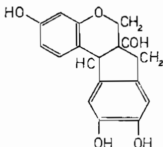
Brasilin
