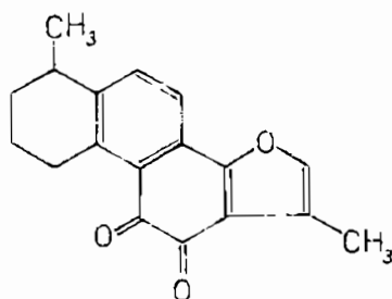
Tansinon I
