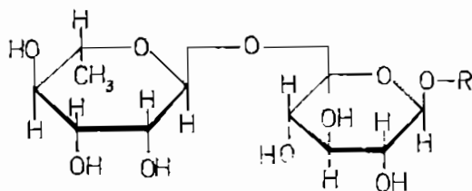
Rutinose
