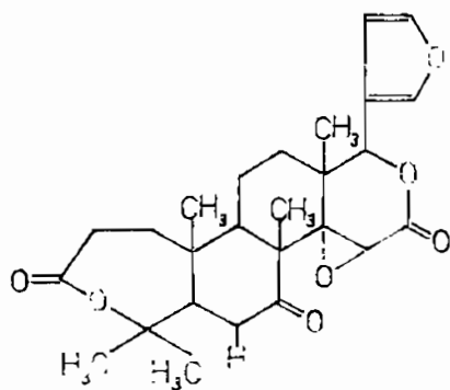
Berberin
